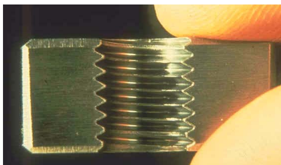
TAPTITE®によって作られたためねじ。
